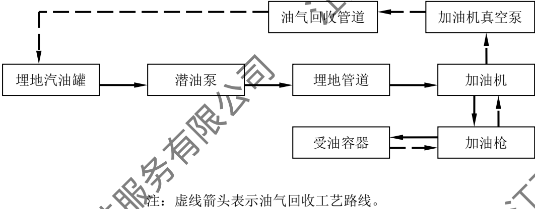
图 2.3-3 汽油加油工艺流程图示意简图
