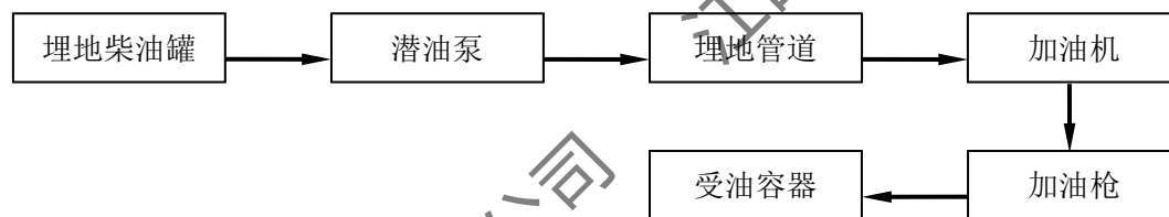
(3) 图 2.3-4 柴油加油工艺流程图示意简图
