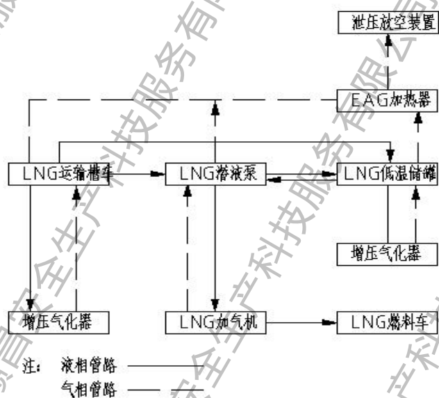
图 2.5-1 LNG 加气流程框图
