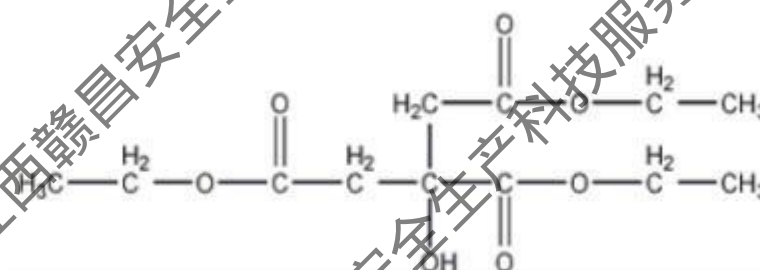
图 2.7-1 松节油结构式
